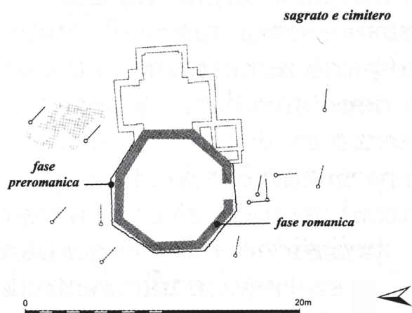
Fig. 13. San Giovanni di Bovolone (Verona), pianta con le due fasi principali della chiesa (da Breda, Manicardi 2002)
