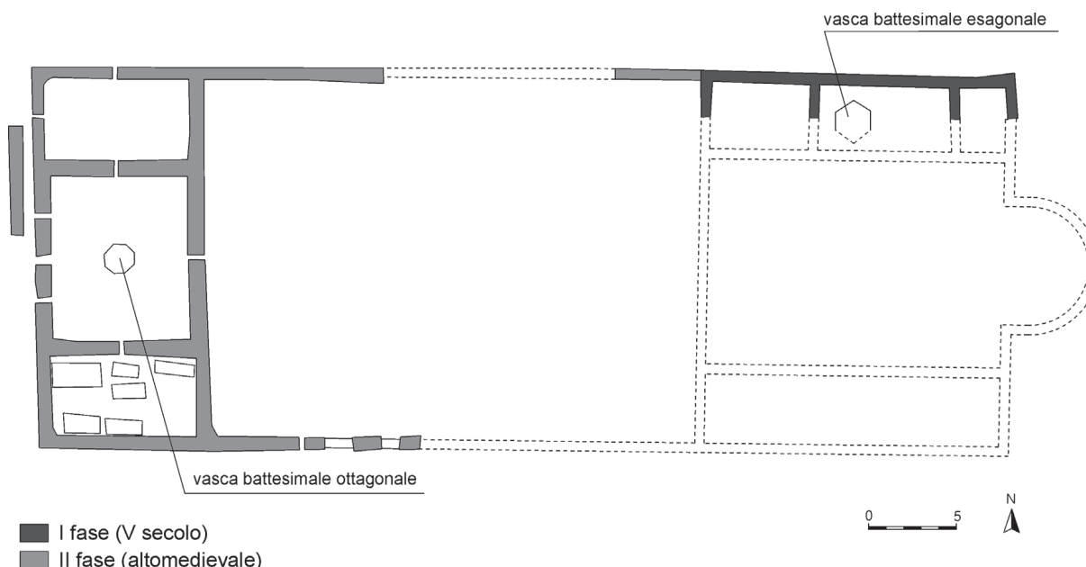
Fig. 17. Santa Maria di Pontenove (Brescia) (da Breda, Venturini 2001)
