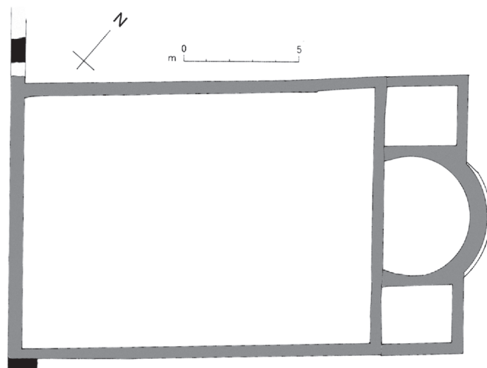
Fig. 1. Sizzano (Piemonte), edificio di culto costruito in una villa funzionante nel V secolo (da Pejrani 2001)
