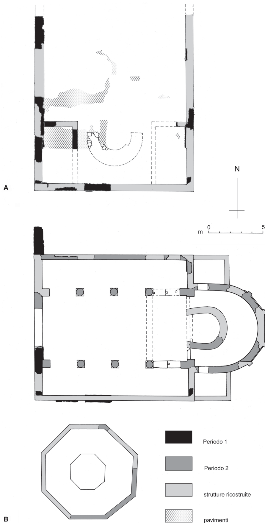
Fig. 2. Pieve di San Vittore di Sizzano. A.-B: 2 fasi dell'edificio di culto (da Pejrani 2001)
