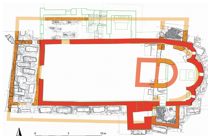
Fig. 7. San Pietro in Mavinas (Sirmione, Brescia), pianta della chiesa con le diverse fasi (per cortesia di A. Breda)
