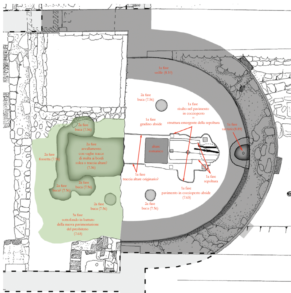
Fig. 3. San Bartolomeo di Bornato (Cazzago, Brescia), fotopiano e disegno dell'abside della chiesa, muri della villa romana e buche di palo dell'insediamento longobardo (per cortesia di A. Breda)
